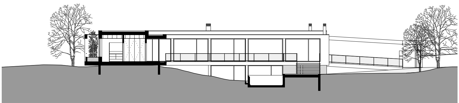
CORTE 04
