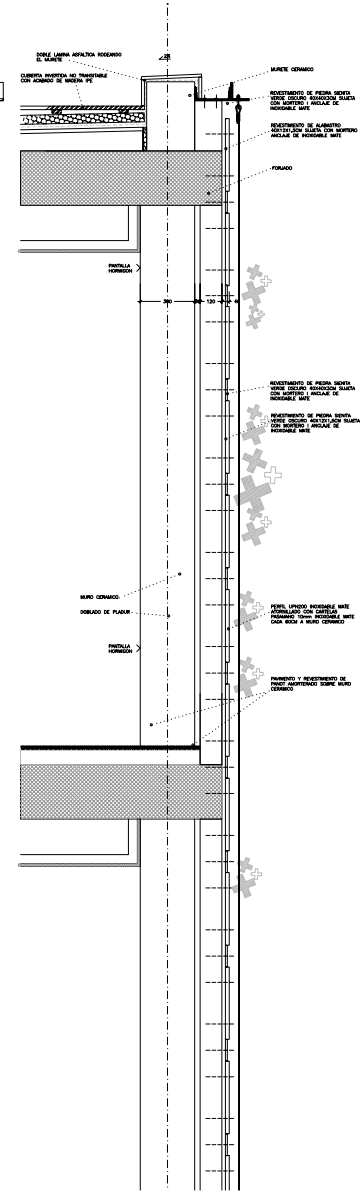
DETALLES FACHADA 0 0.5 1 2 3
