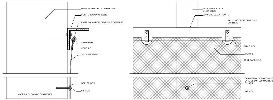
DETAIL B | ECH. : 1/5 FIXATION DE LA TOILE PARE-VENT FIXATION PAR PATTE GALVA BOULONNEE SUR LA CORNIERE ESPACEMENT 225 MM FIXATION SUR LES MADRIERS PAR DES OERLETTES ET VIS
