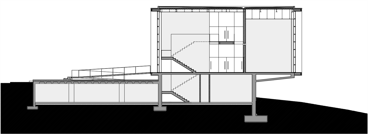
Corte C7
