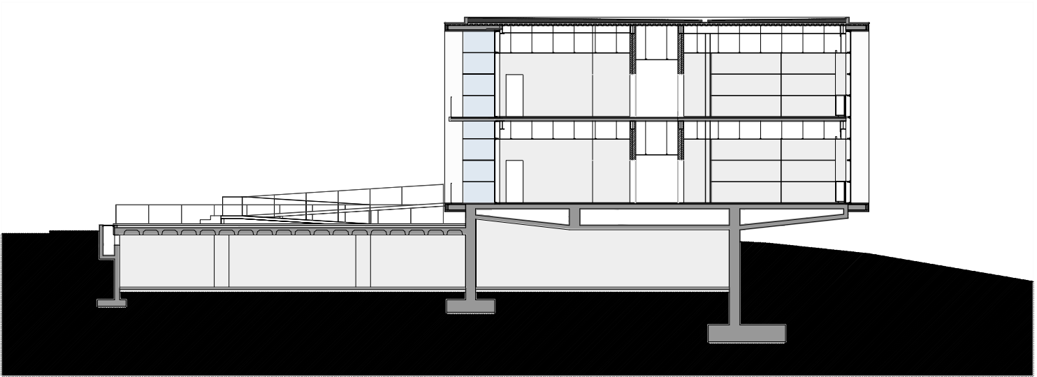
Corte C5
