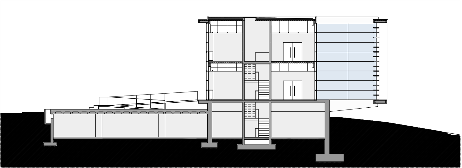
Corte C6
