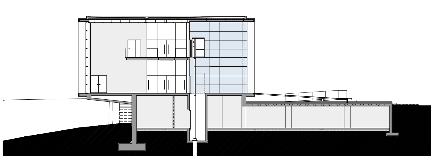
Corte C4
