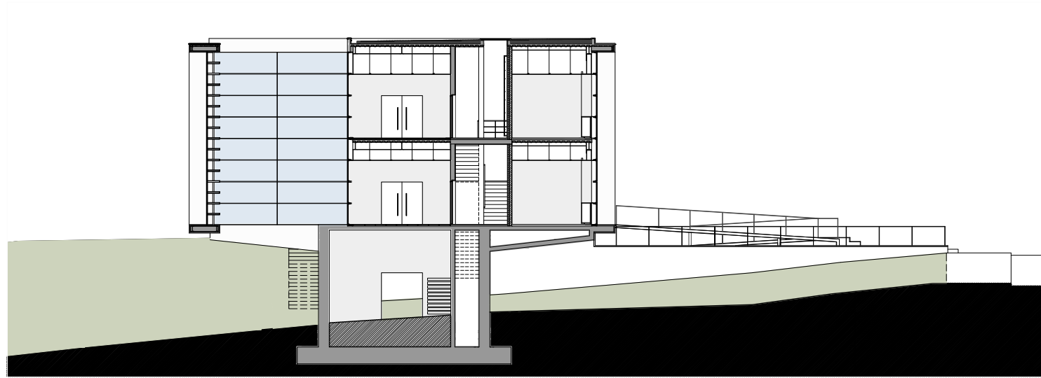
Corte C2
