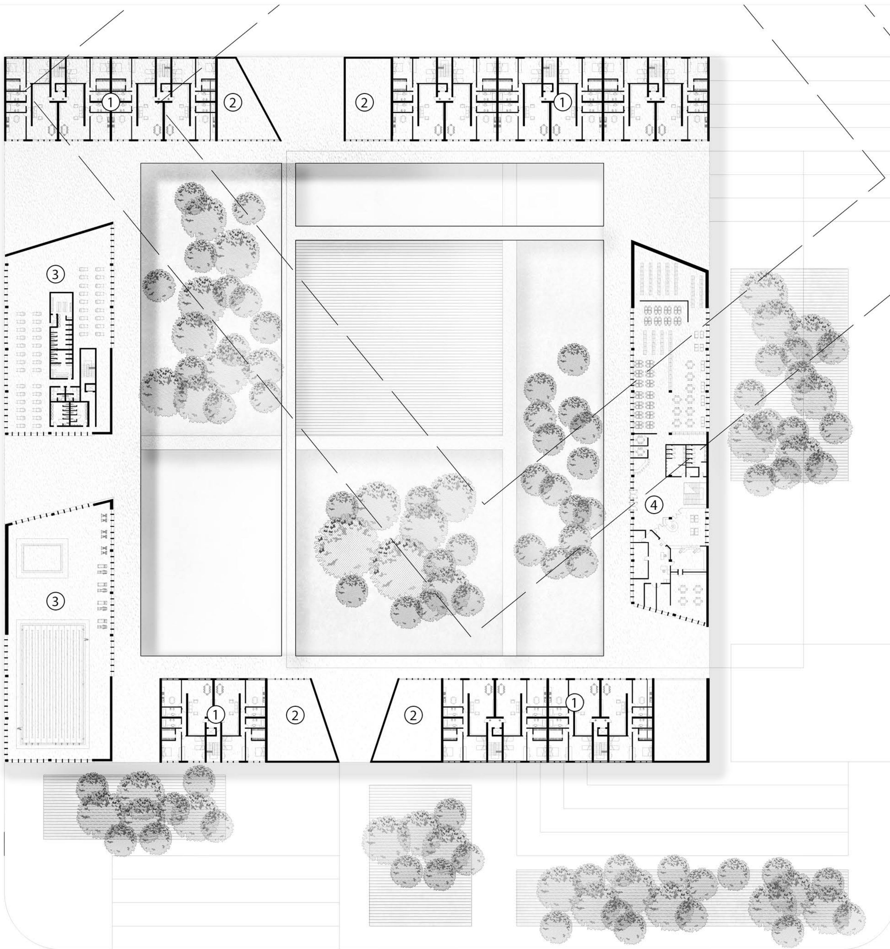
Rap. 1:500 Pianta e Sezione tipo
