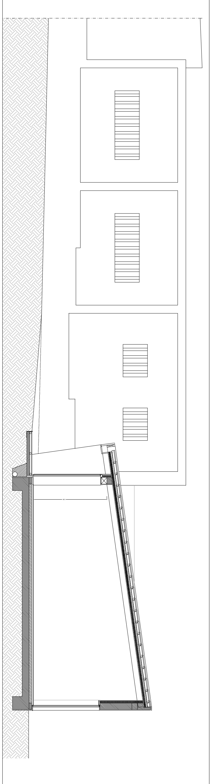
Corte 1
