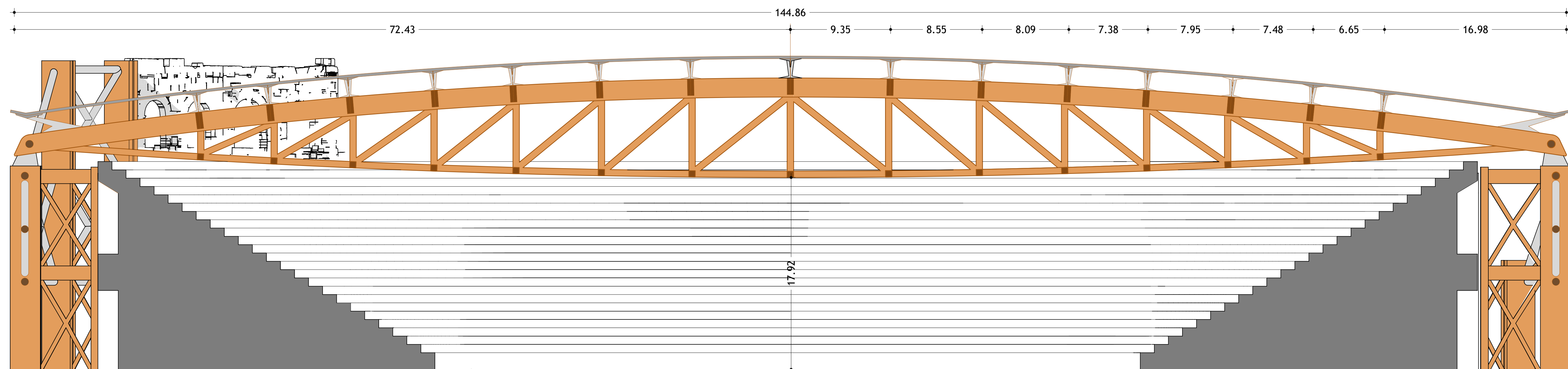
SEZIONE LONGITUDINALE 1:200
