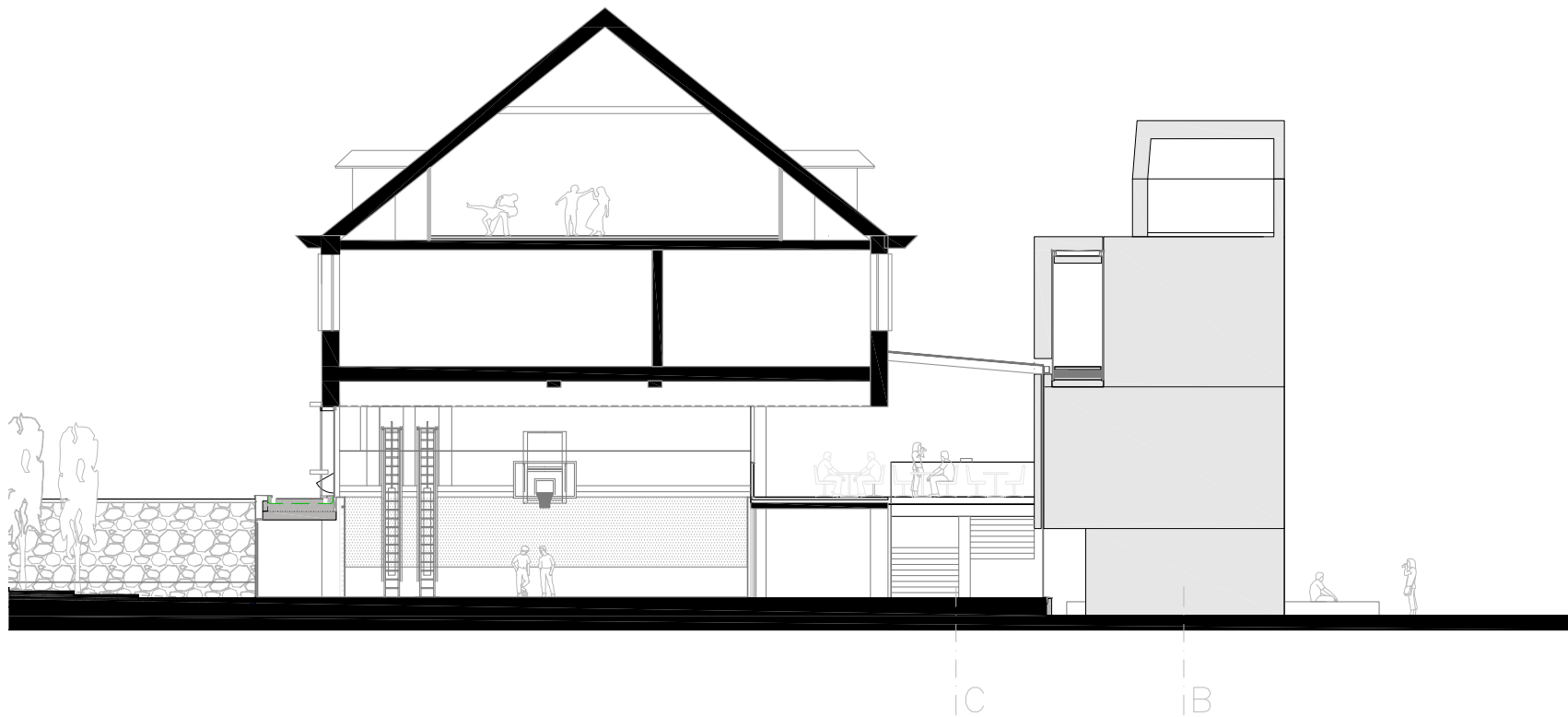
0 1 5 ansicht nordwest schnitt c [1:200] hs rattenberg
