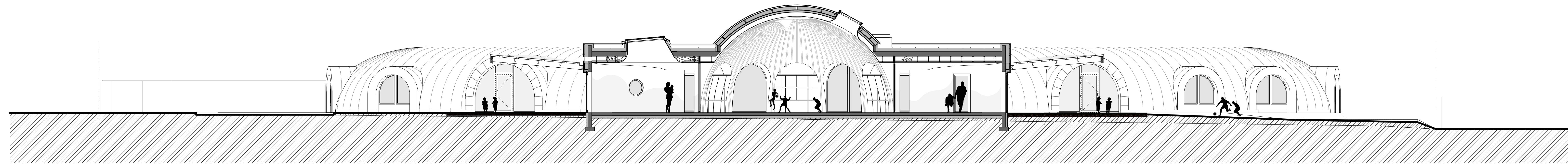
COUPE AA
