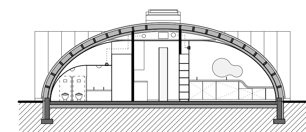
COUPE EE
