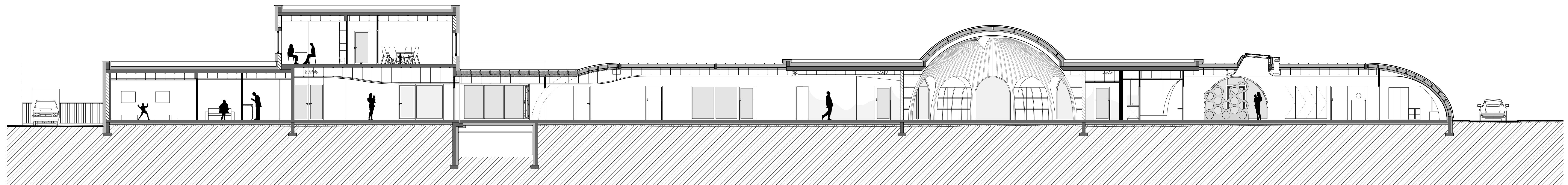
COUPE BB
