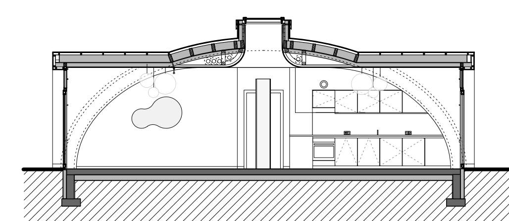
COUPE DD
