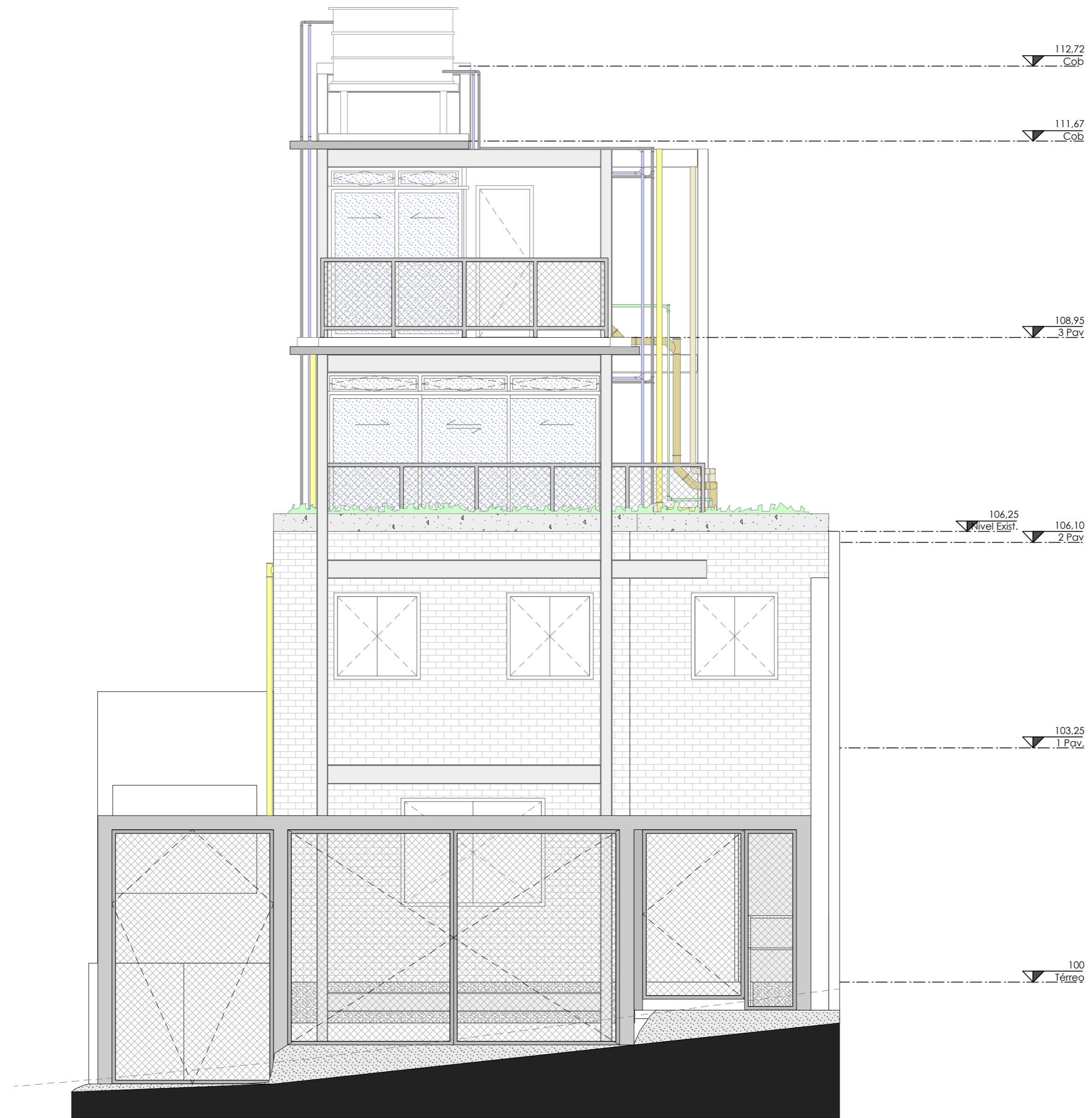
ELEVAÇÃO FRONTAL
