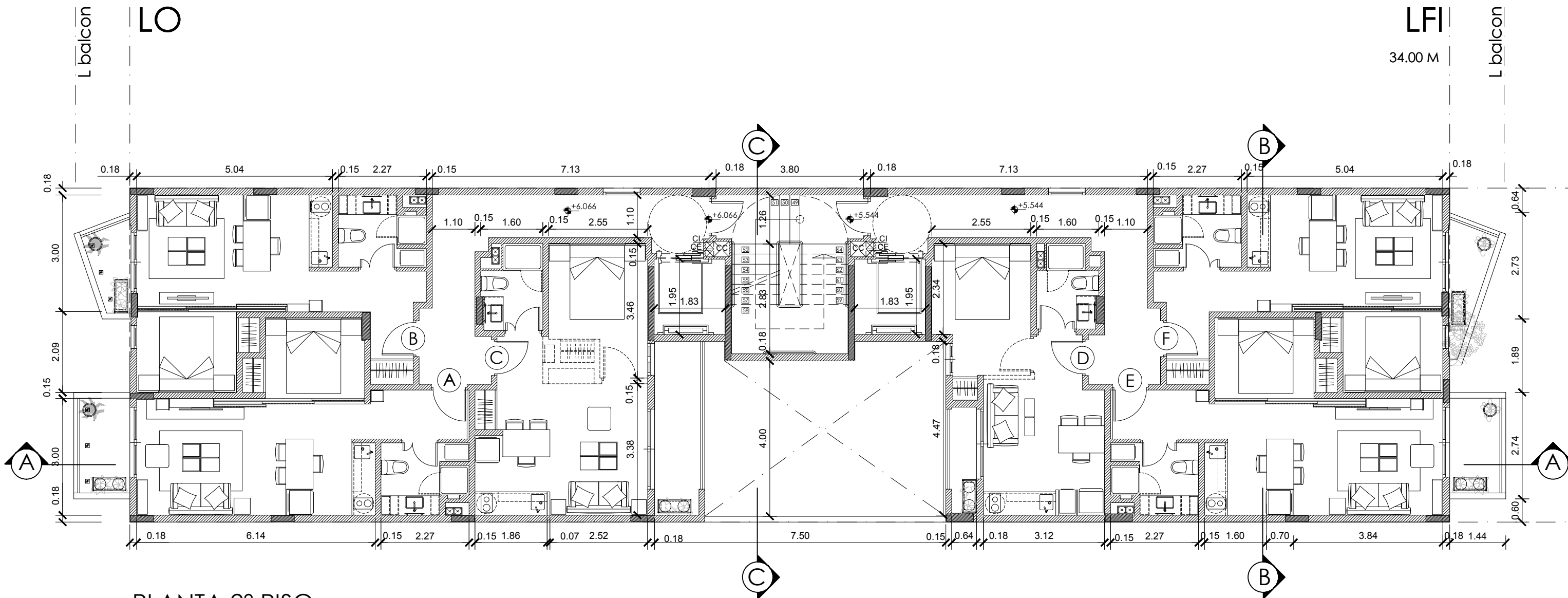
PLANTA 2° PISO
