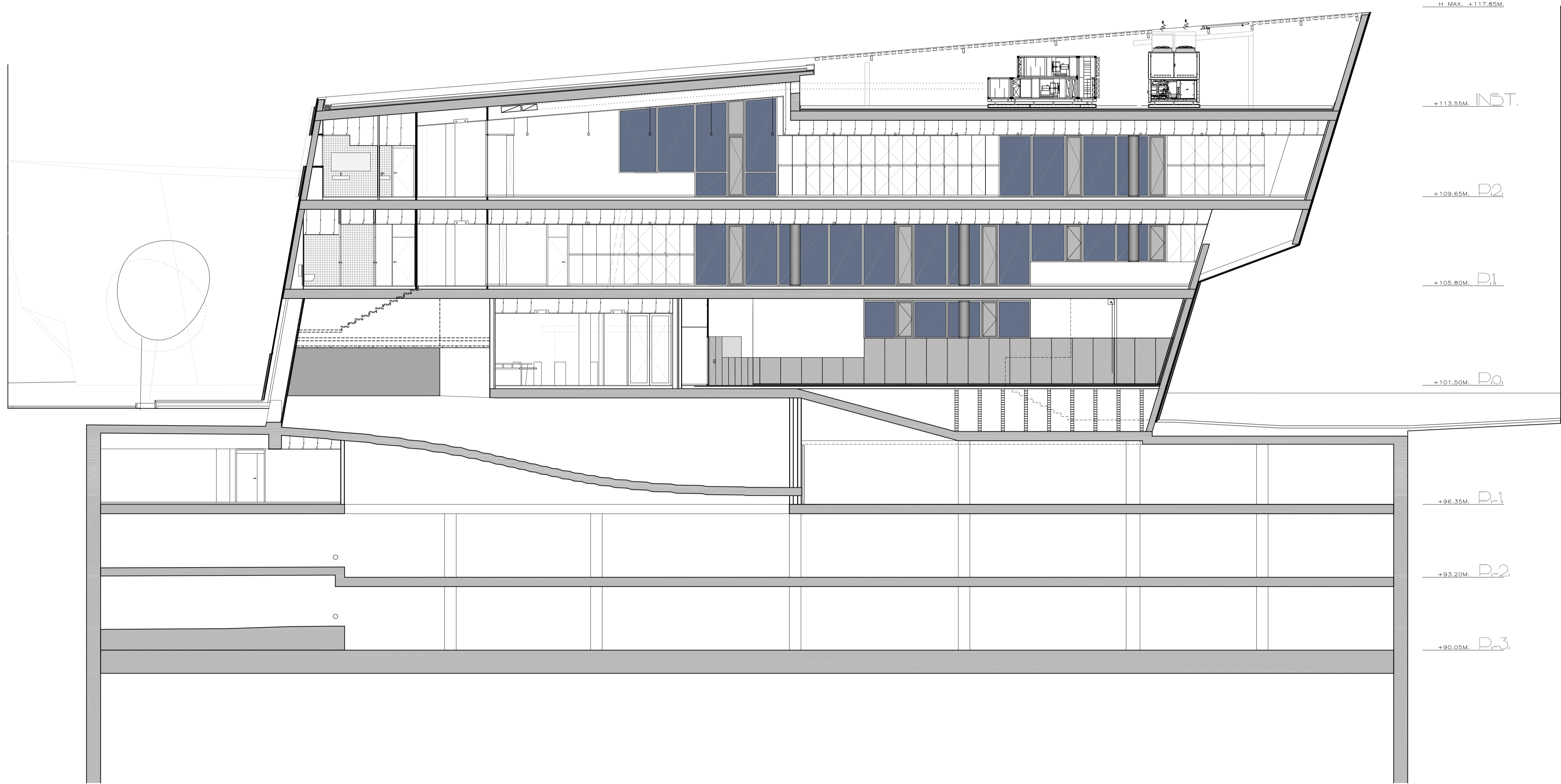
SECCIÓN LONGITUDINAL
