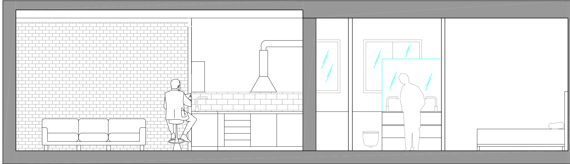
Sección FF'
