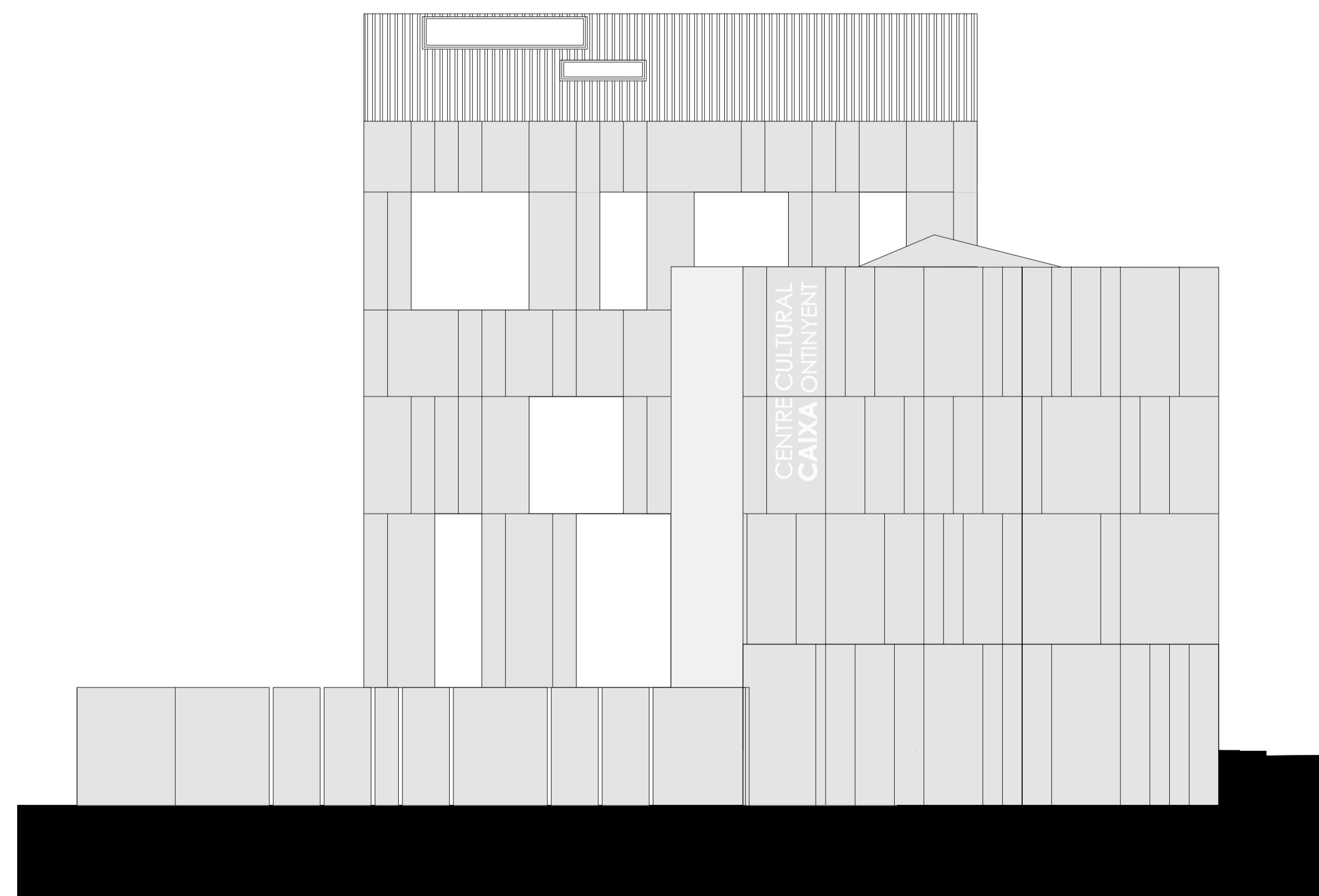
ALZADO NOROESTE 0 5
