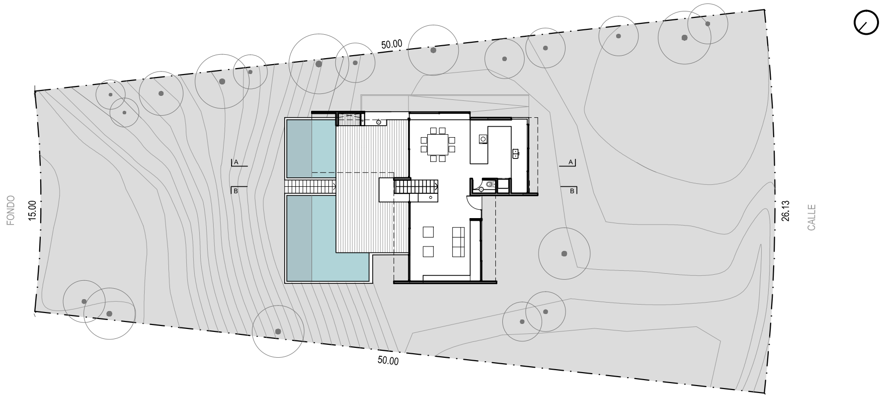
CASA VP - PLANTA PRINCIPAL
