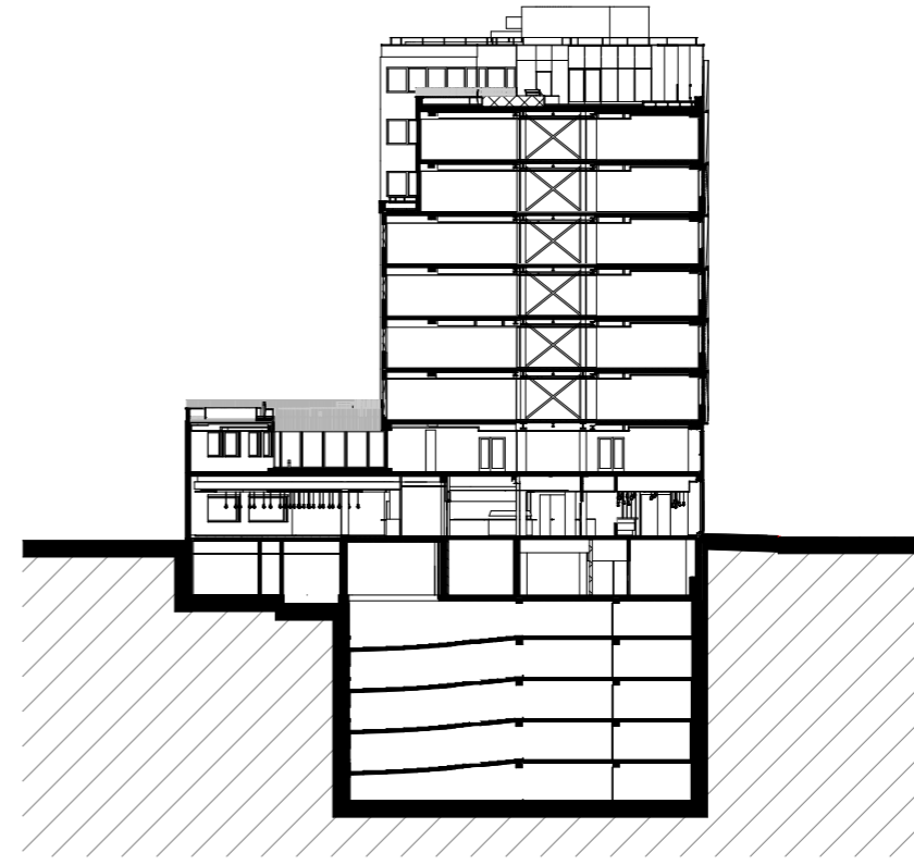
Coupe BB
