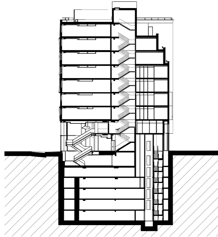
Coupe AA
