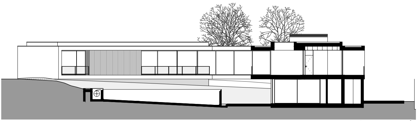
CORTE 01
