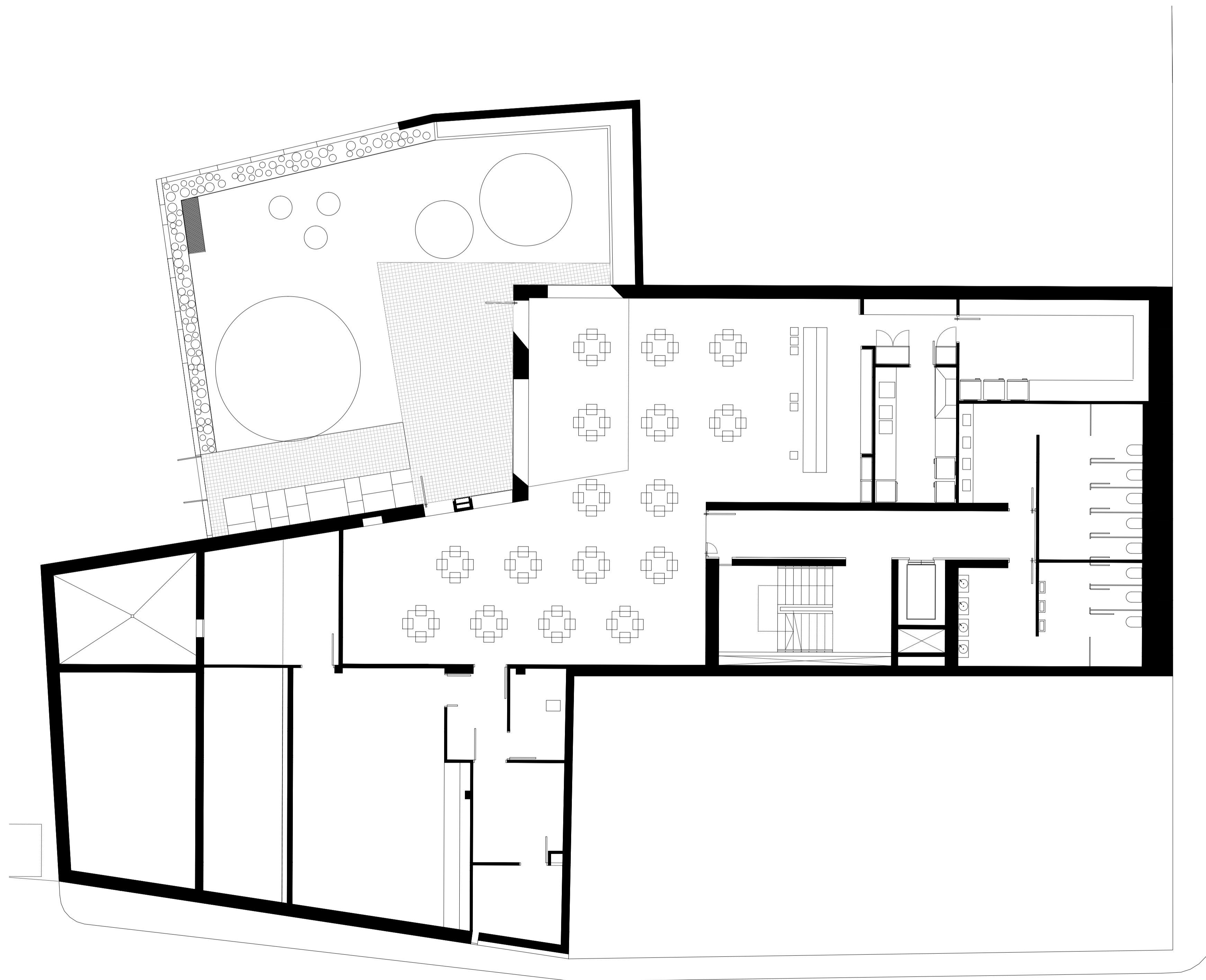
PLANTA SÓTANO 0 5
