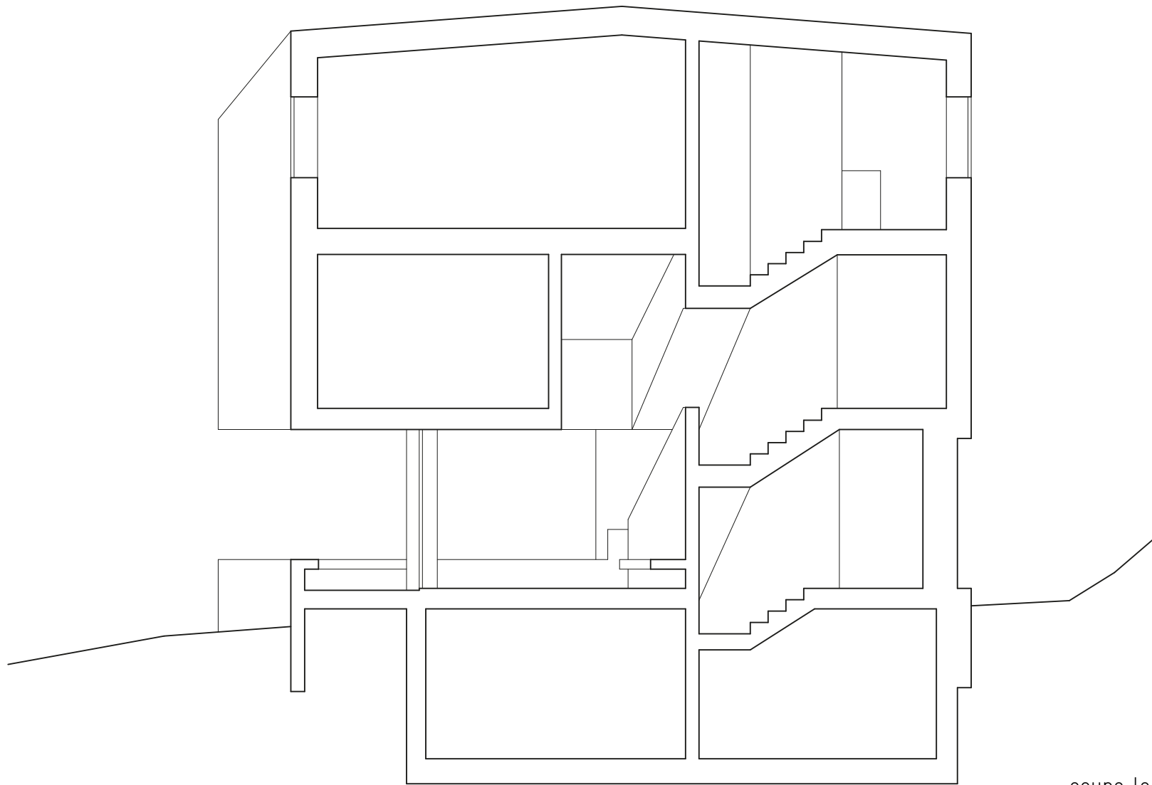
coupe longitudinale
