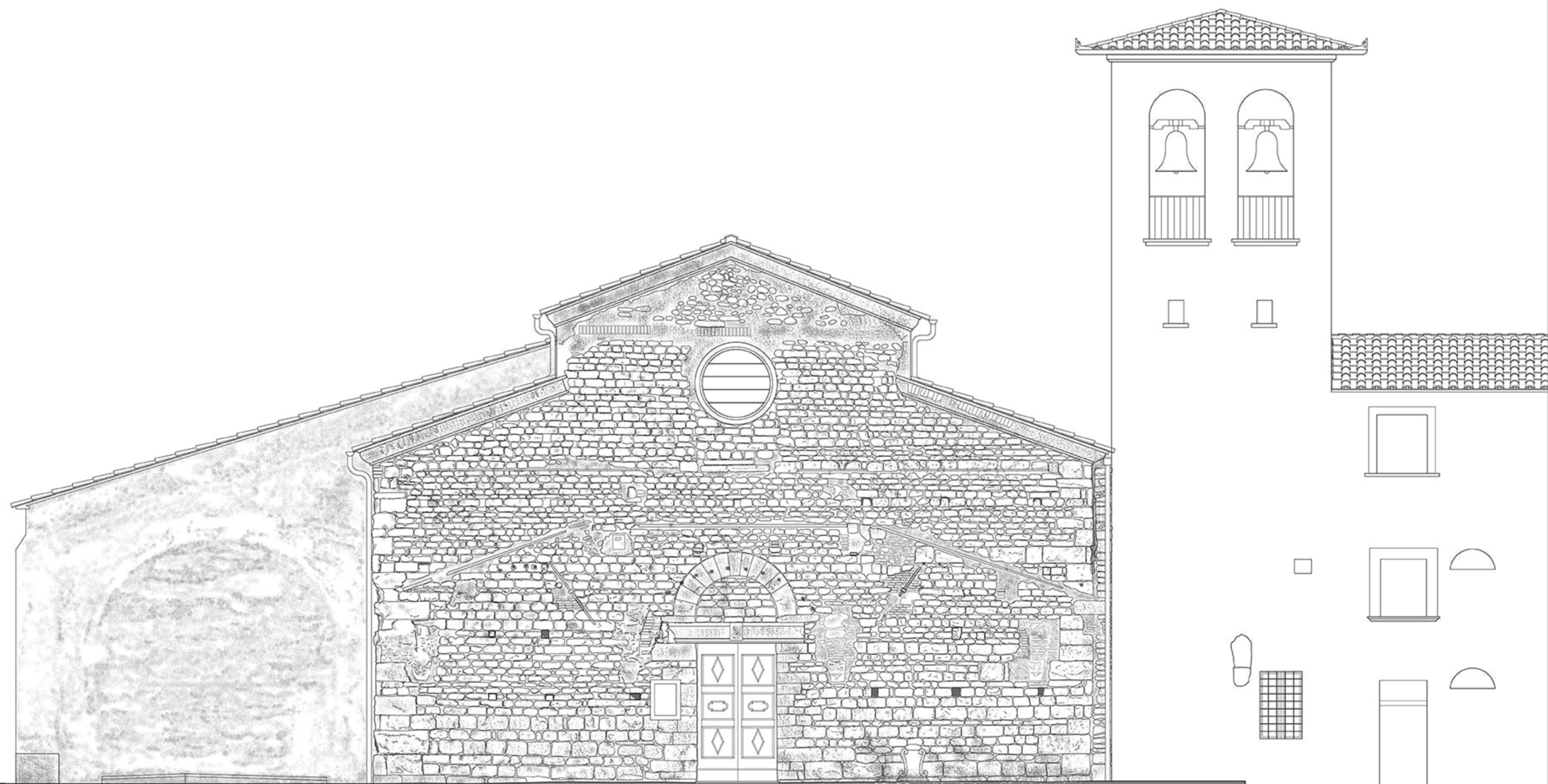
PROSPETTO OVEST
