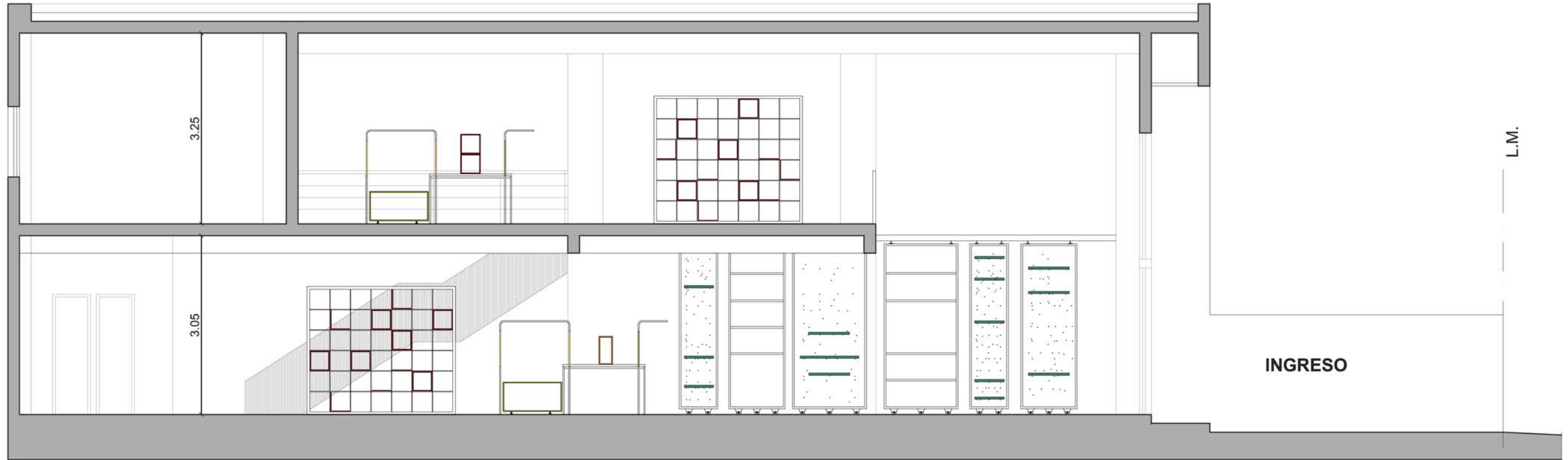
CORTE LONGITUDINAL 2 - OPCIÓN DE CONFIGURACIÓN E. 1:75
