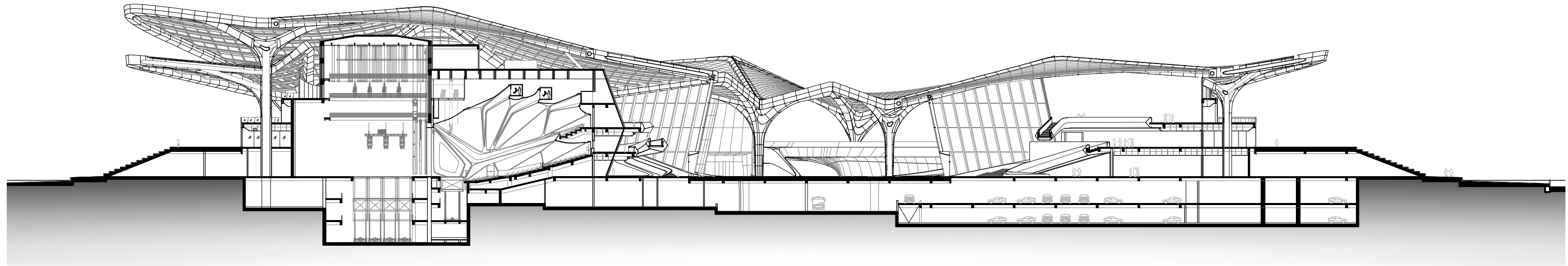
1 SECTION AA' Scale: 1/800
