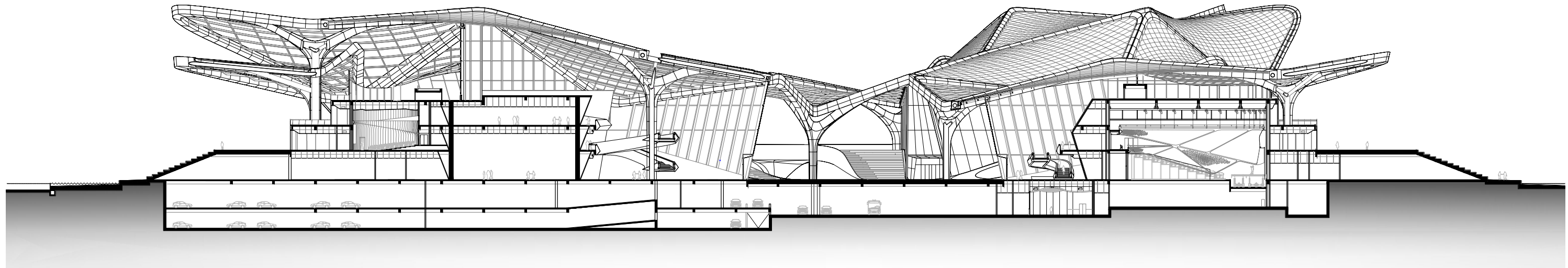
2 SECTION BB' Scale: 1/800
