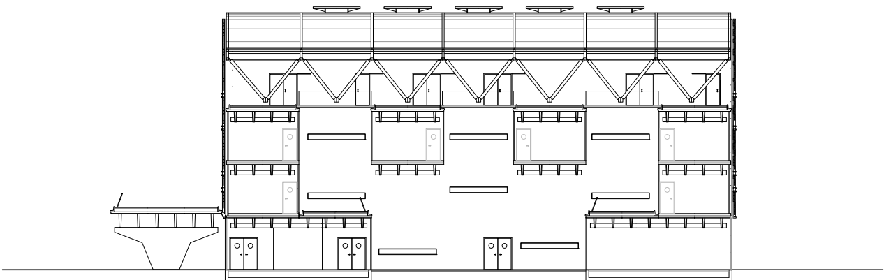
Seccion Longitudinal
