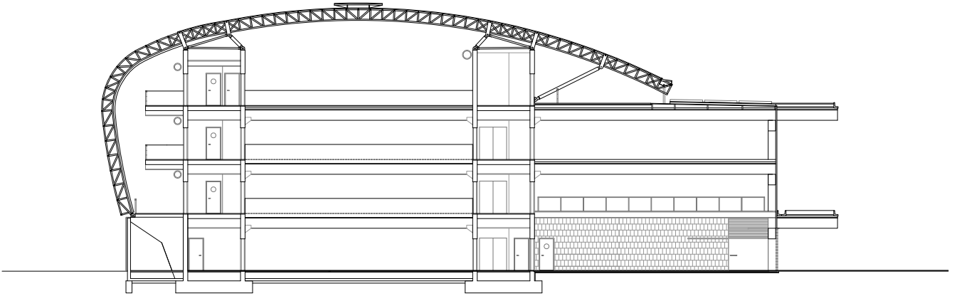
Seccion Transversal
