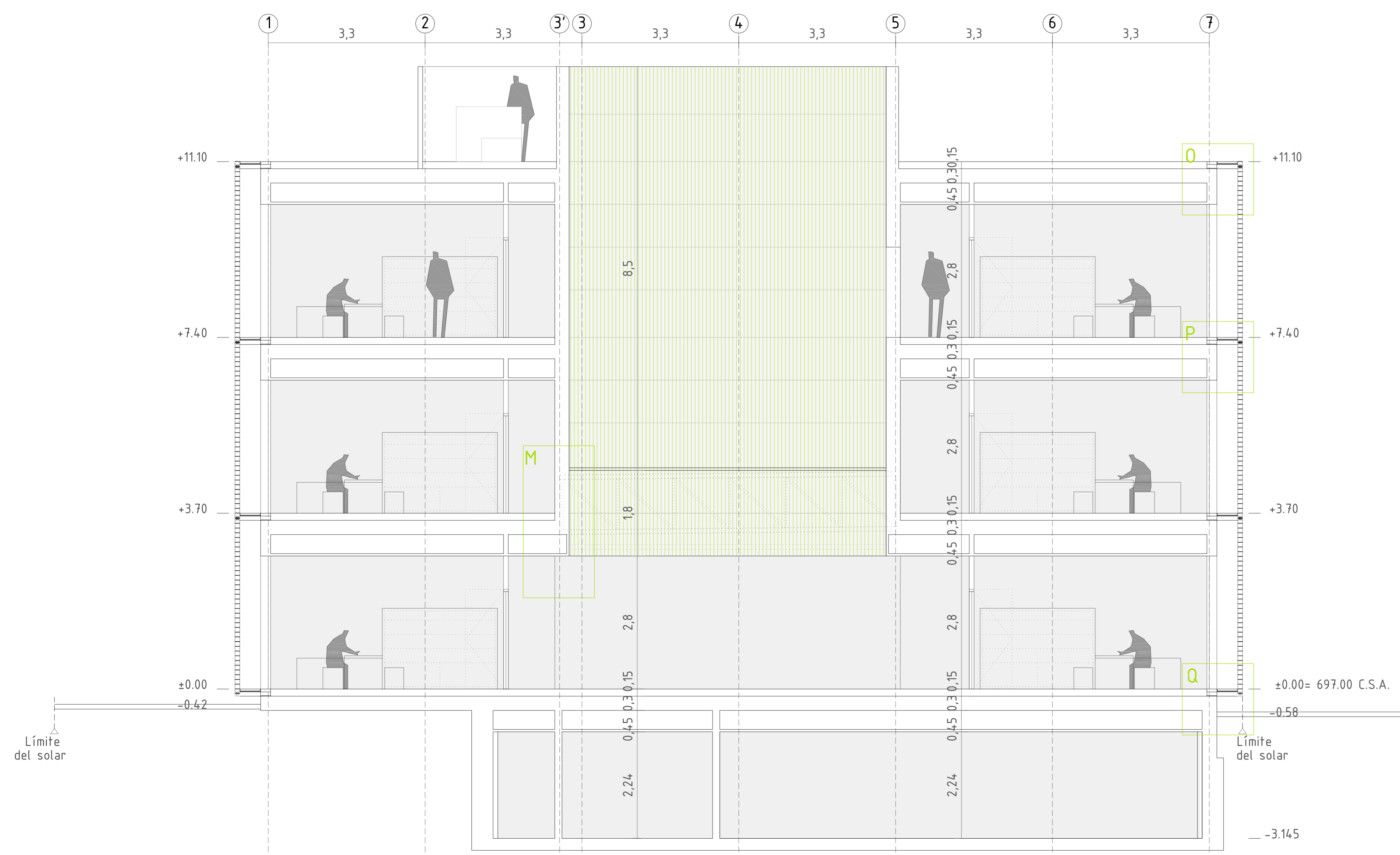
SECCION TRANSVERSAL 1
