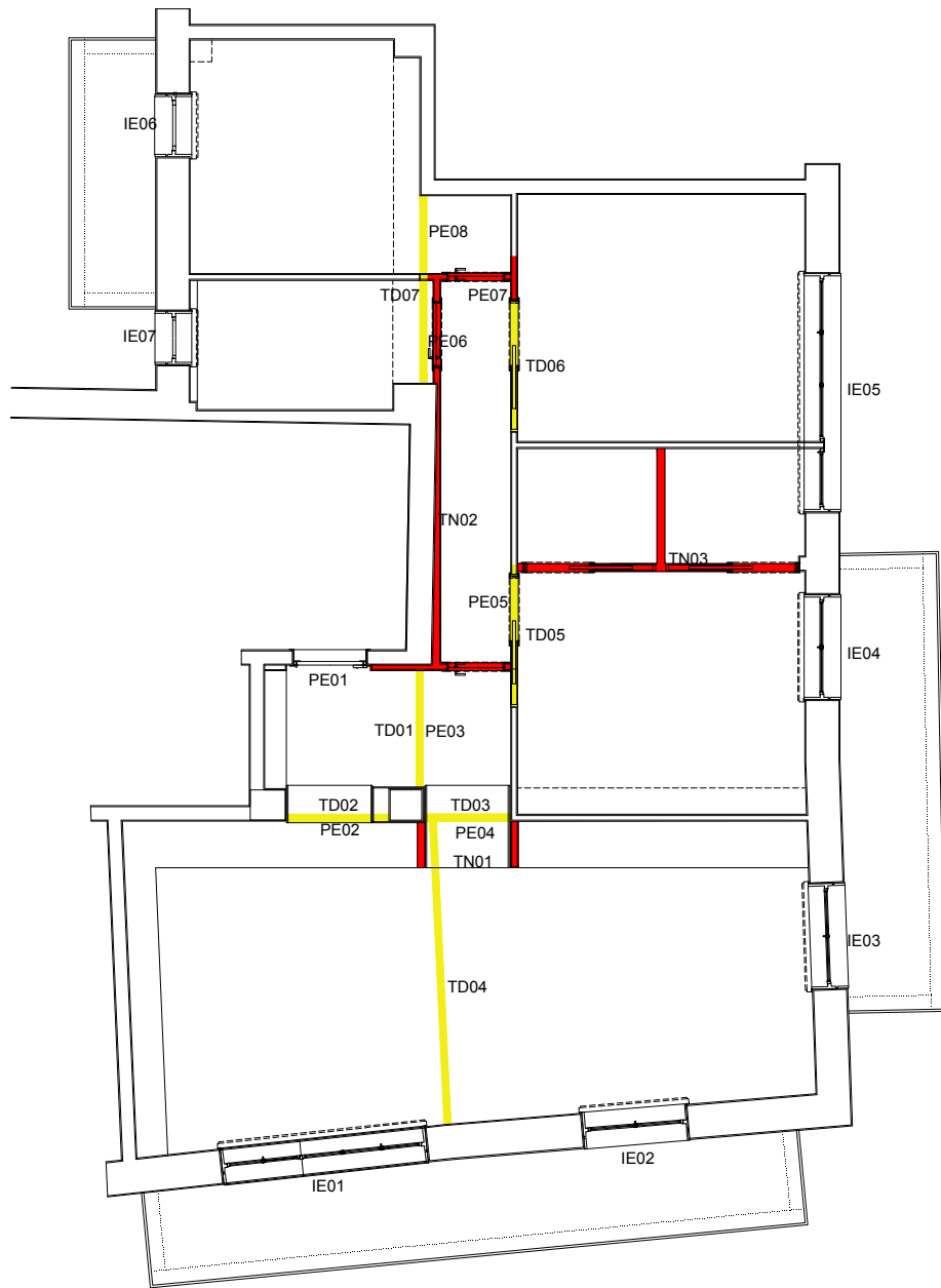
Pianta Demolizioni e Nuovi tramezzi | scala 1:100
