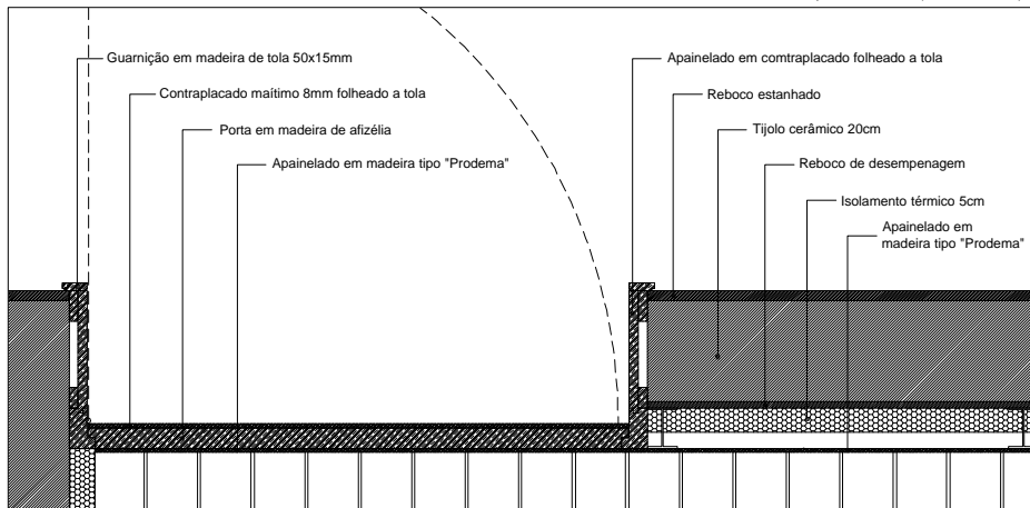
Pormenor de porta de entrada (corte Horizontal)
