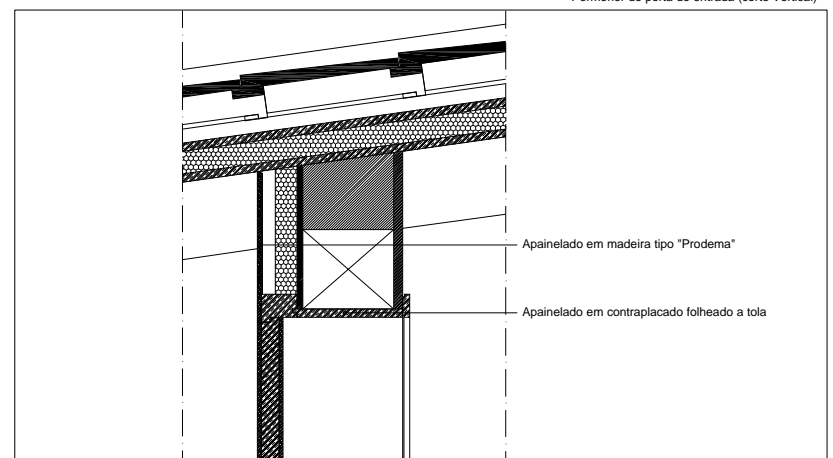
Pormenor de porta de entrada (corte Vertical)
