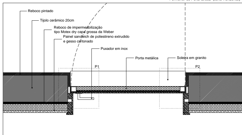
Pormenor de porta de entrada (corte Horizontal)
