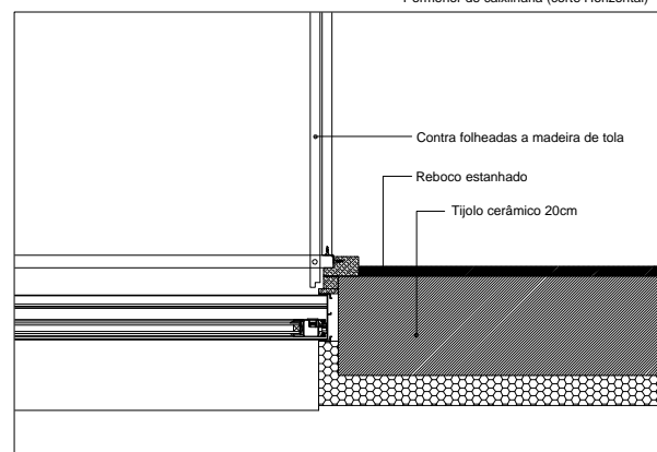
Pormenor de caixilharia (corte Horizontal)
