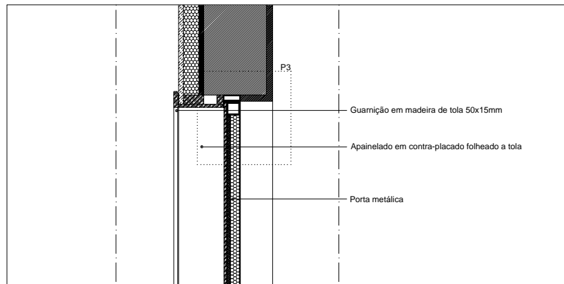
Pormenor de Porta tardoiz (corte vertical)
