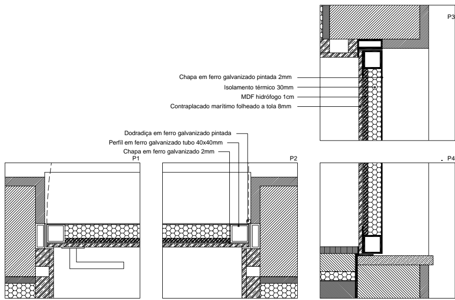
Pormenor de Porta tardoiz (corte vertical)
