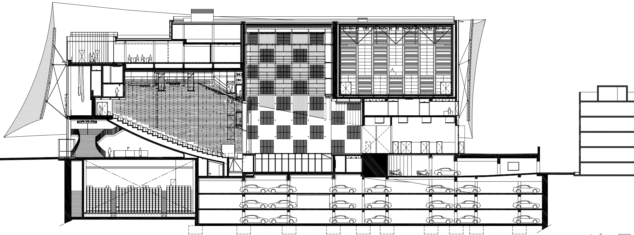
COUPE LONGITUDINALE AA
