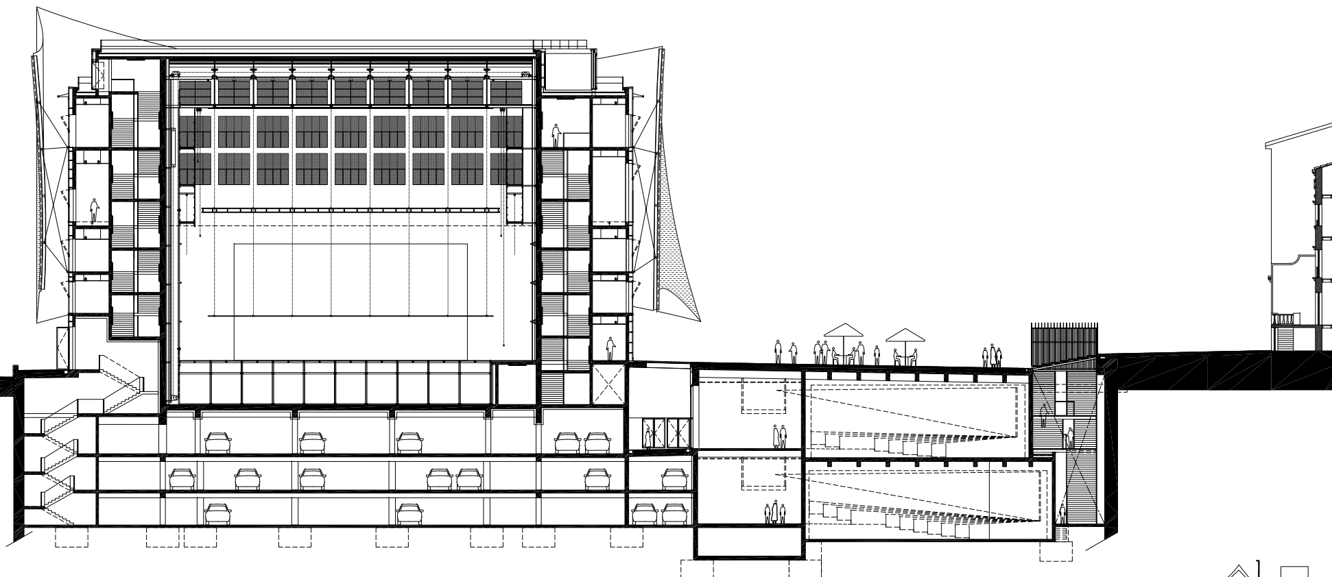
COUPE TRANSVERSALE CC
