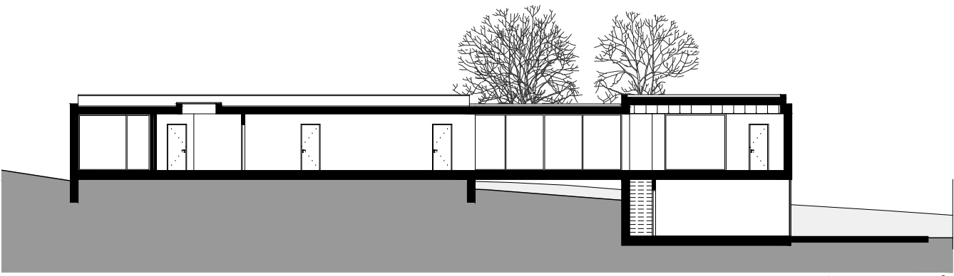
CORTE 03
