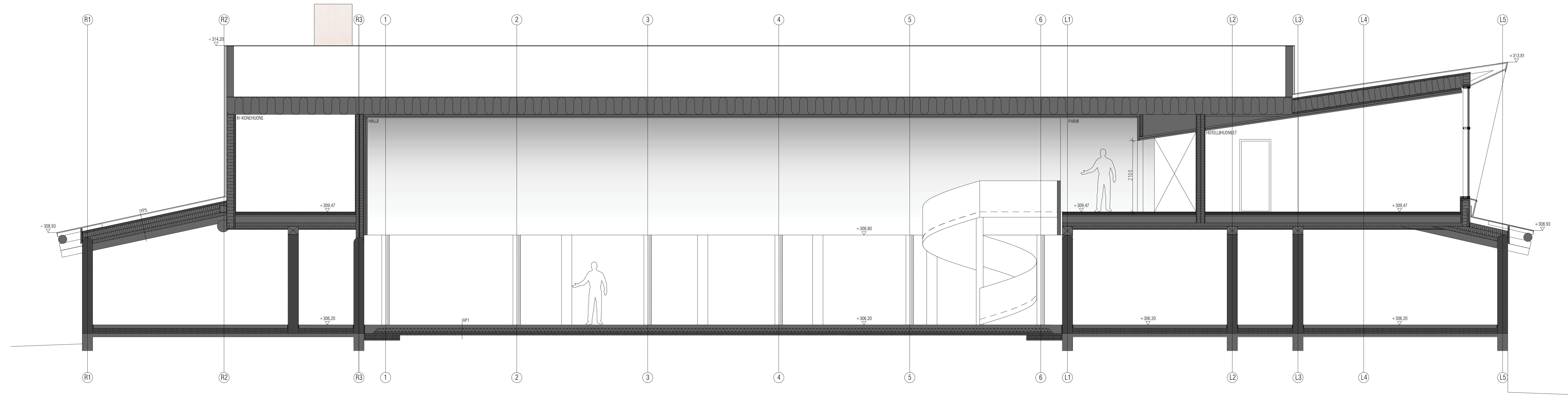
Leikkaus A-A / 1:50
