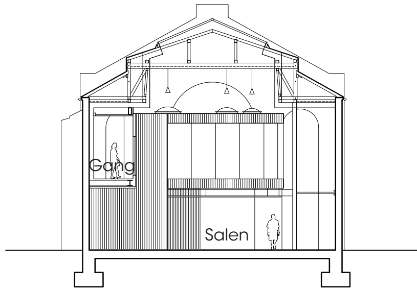
snit B-B 1:200
