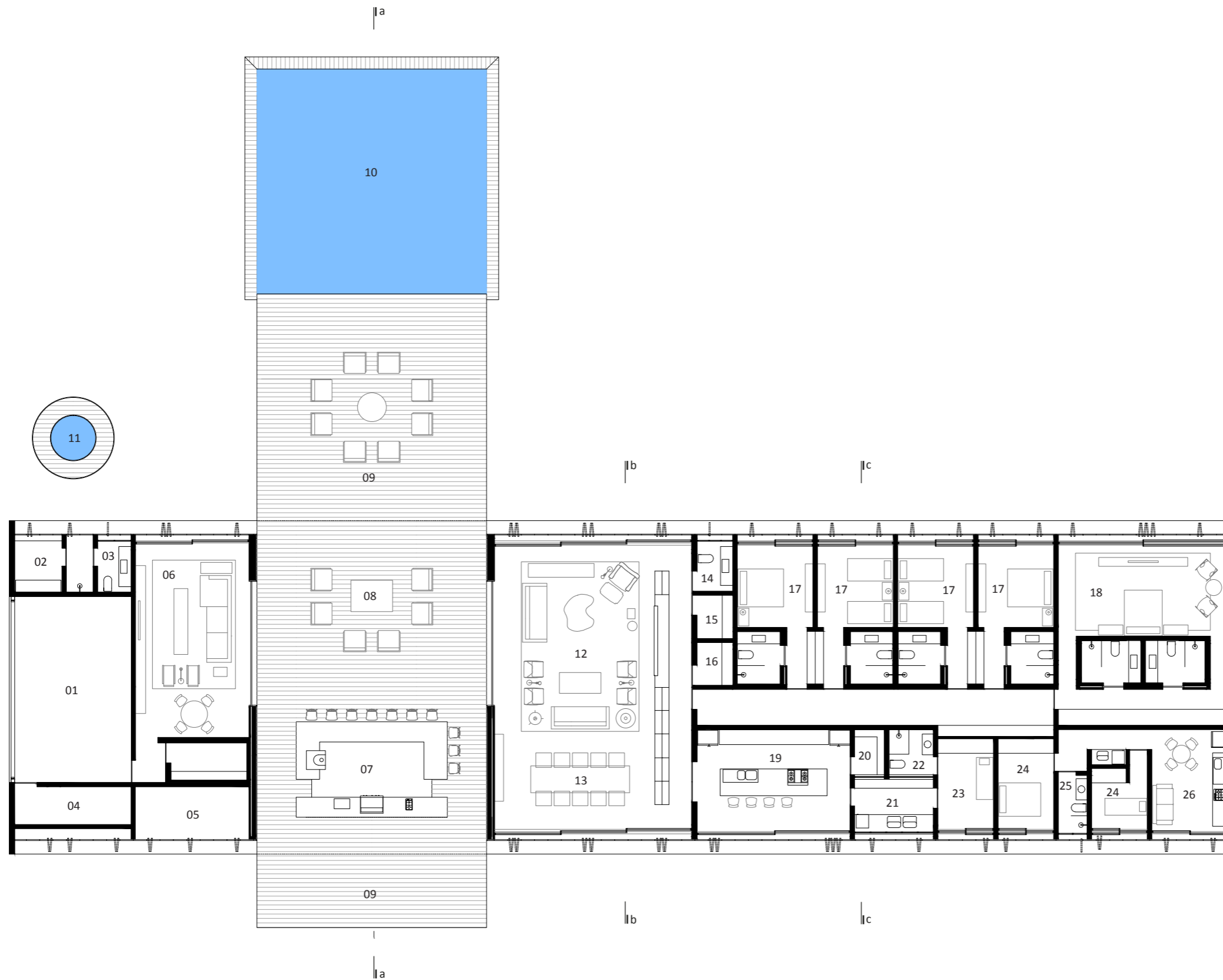
planta térreo _ groundfloor
