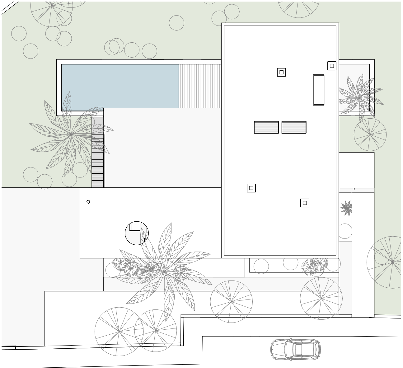
PLANTA COBERTURA
