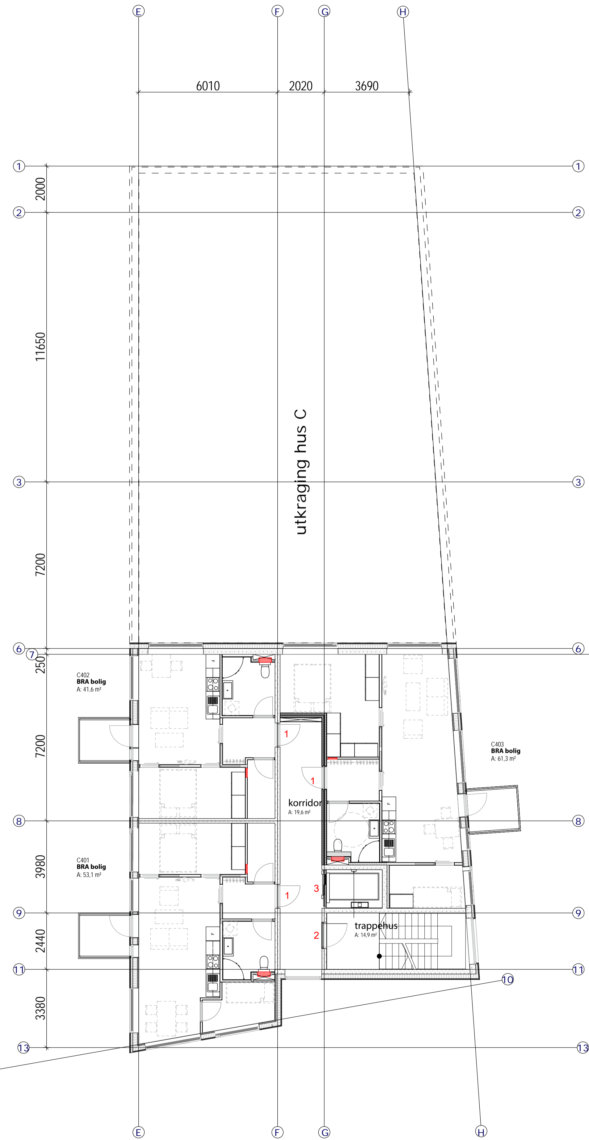
hus C plan 4 Støperiet 4.etasje Dato: 18.10.2013
