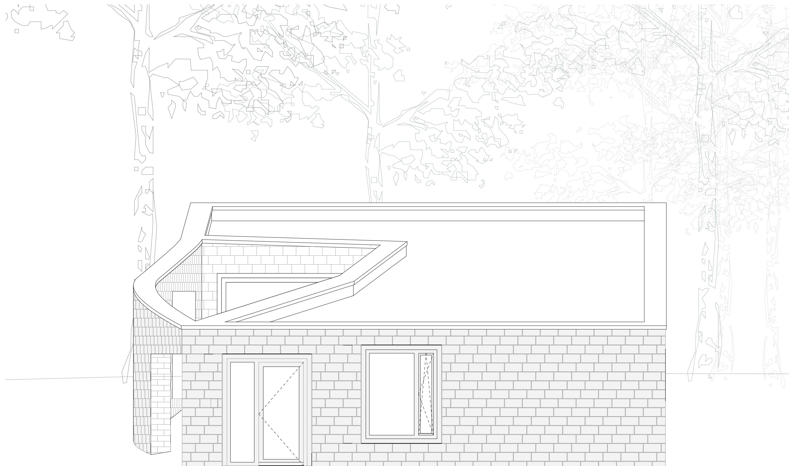
aanzicht voorgevel - schaal 1/50
