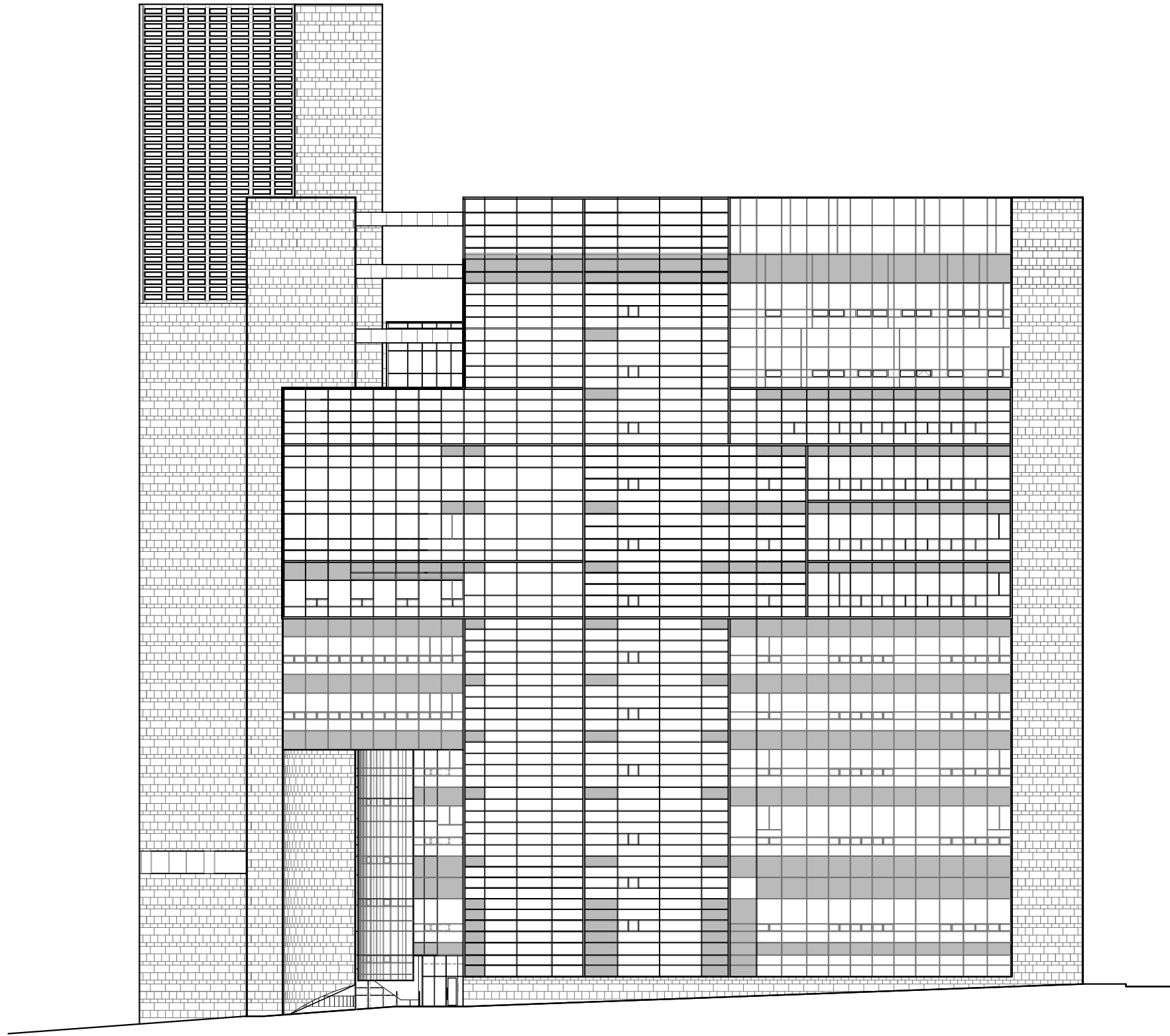
1 우측면도 1/400
