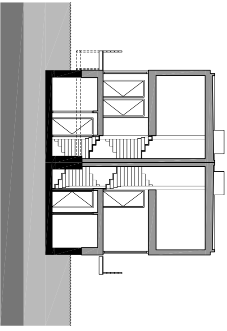
doorsnede B
