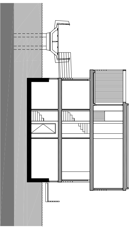
doorsnede A
