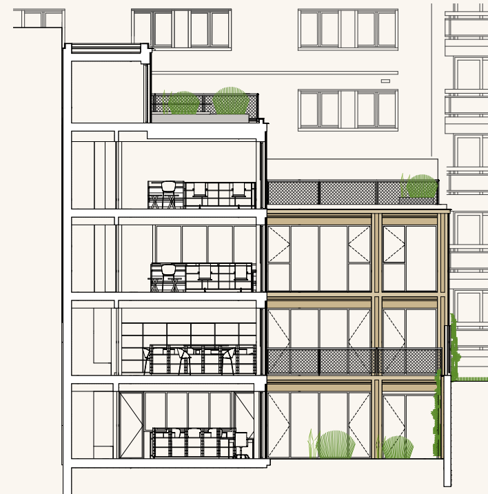
Coupe transversale
