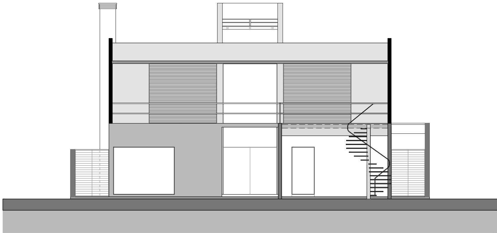
FACHADA POSTERIOR
