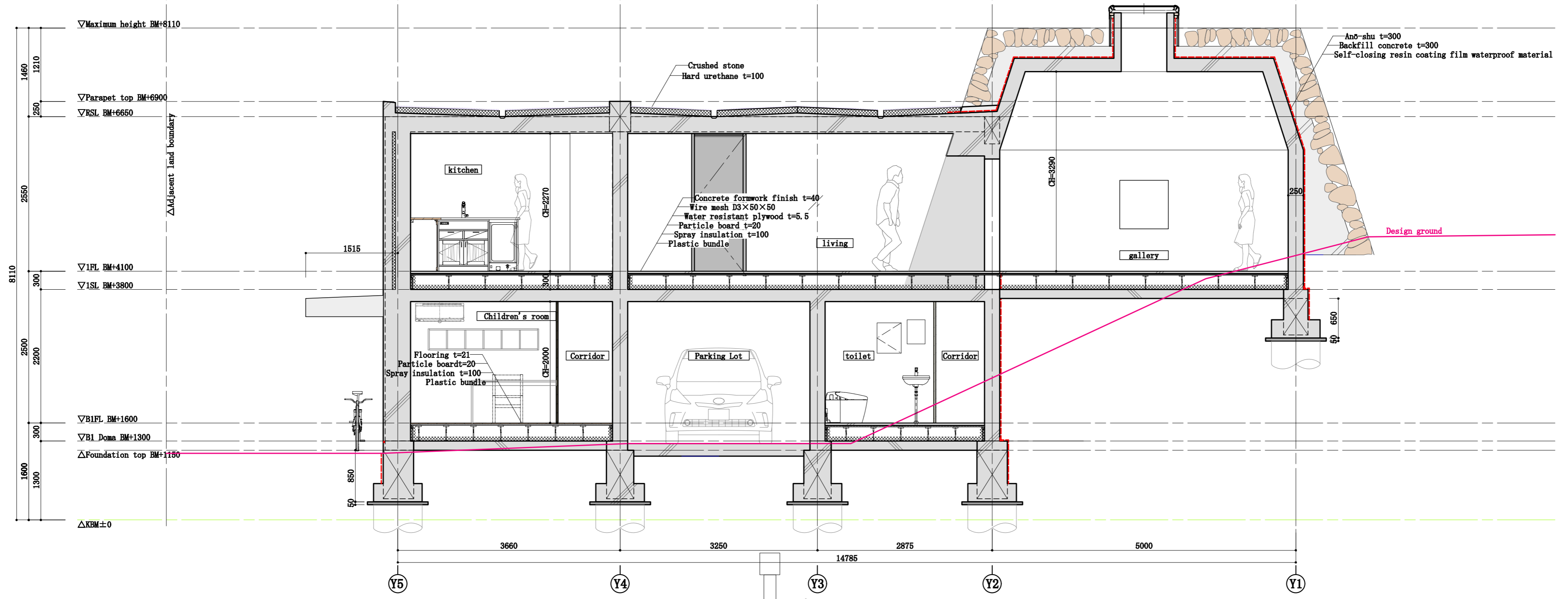
A-A' Section
