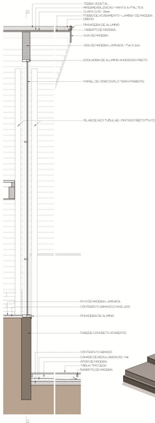
CORTE DE PELE 1:20
