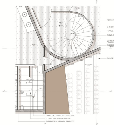
AUDITORIO AMPLIADO 2 1:20
