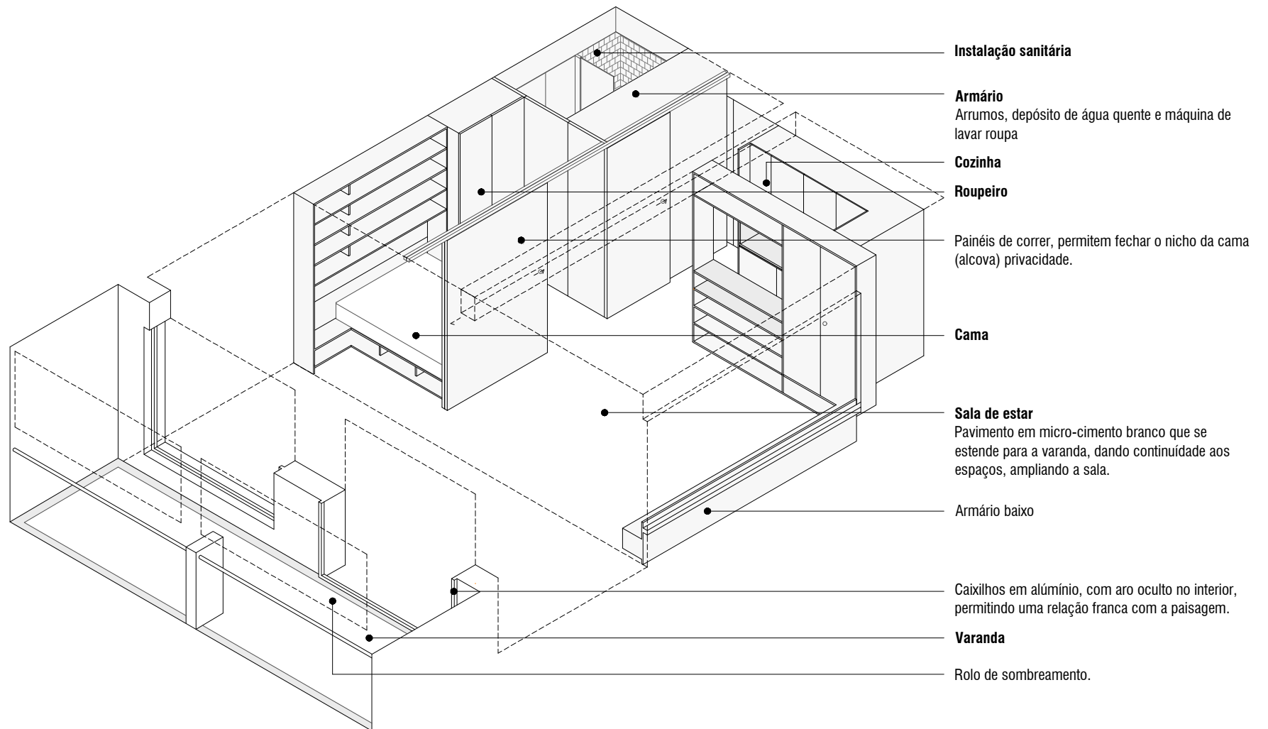
Axonometria
