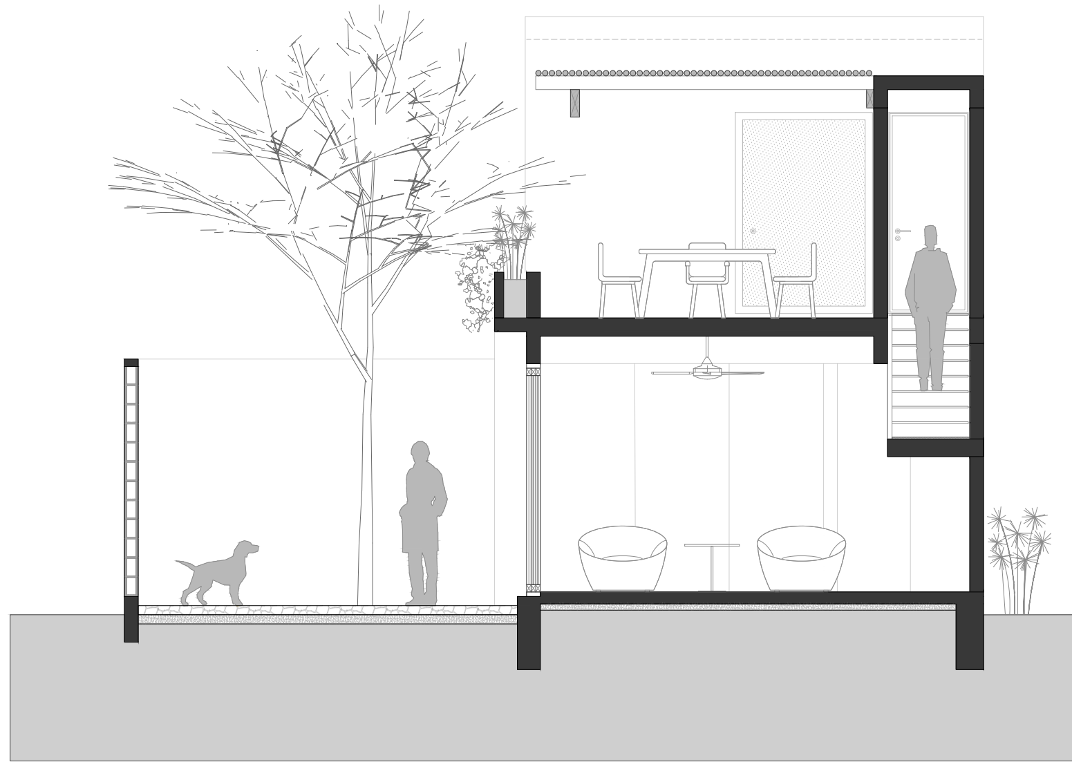
Villa 03 | Corte D-D'
