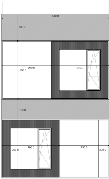
ALZADO B
