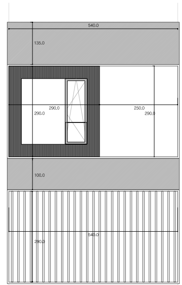
ALZADO D
