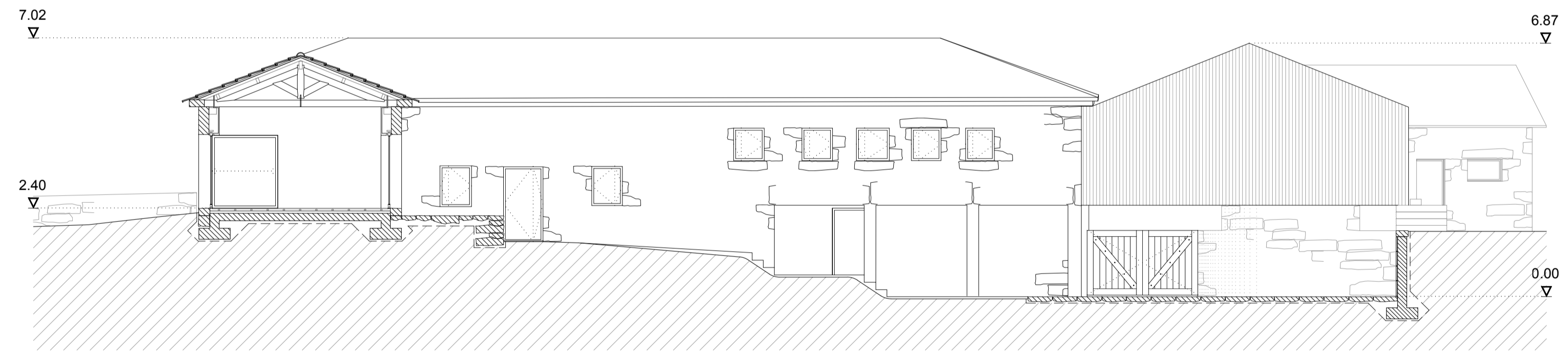
CORTE TRANSVERSAL 01
