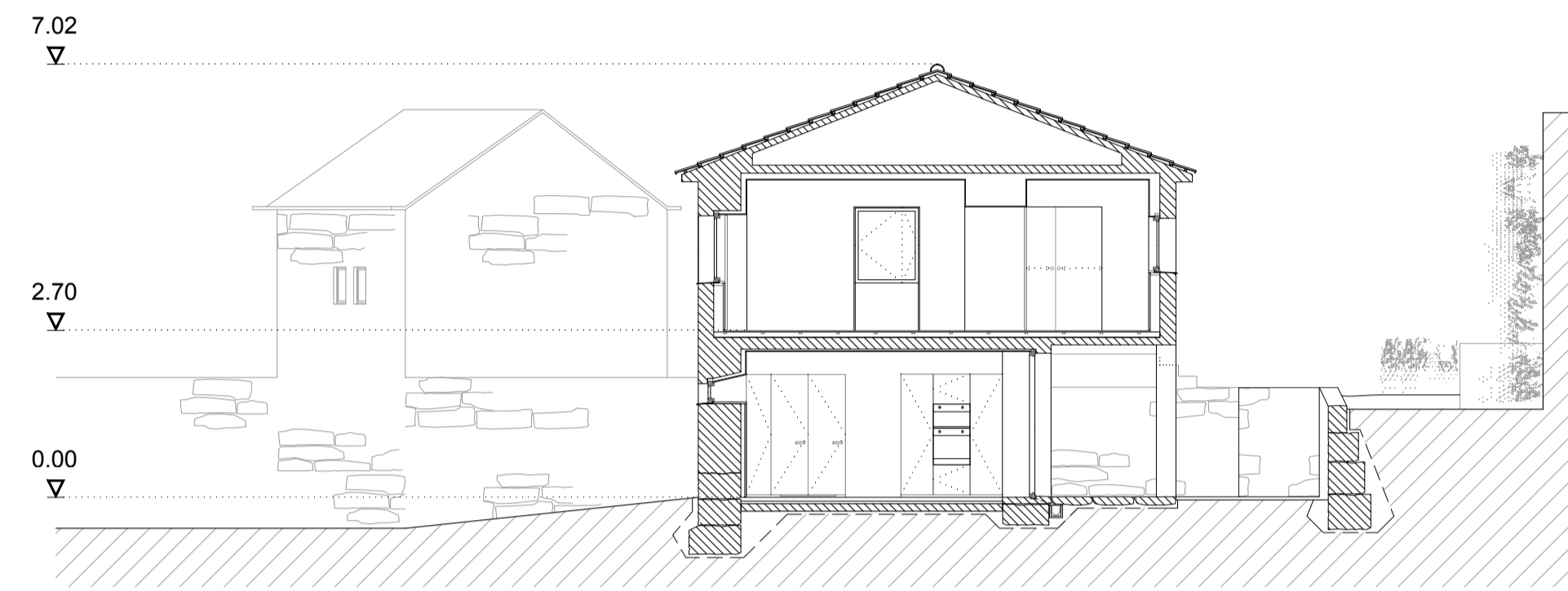
CORTE TRANSVERSAL 03
