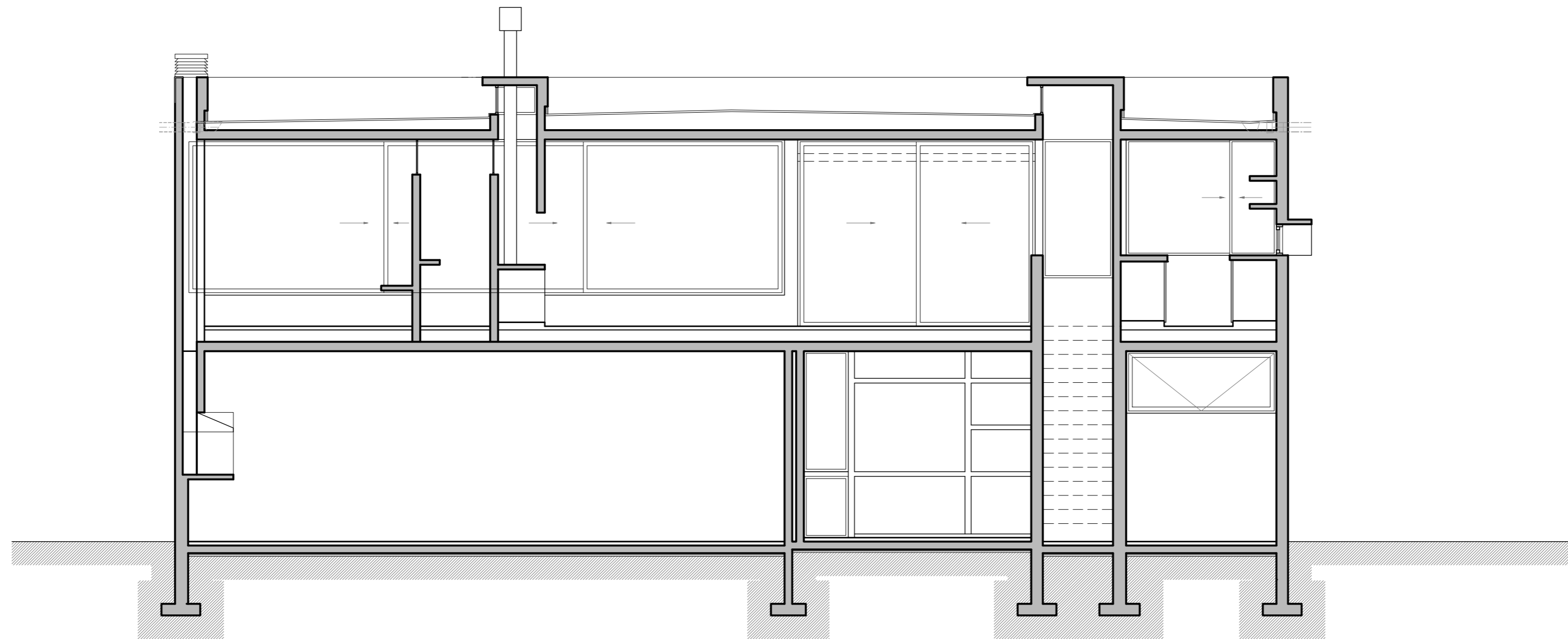
CORTE 2-2
