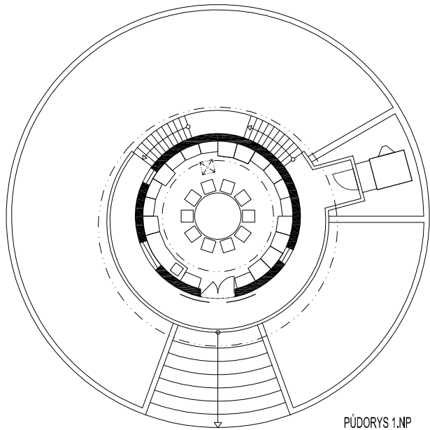
PŮDORYS 1.NP
