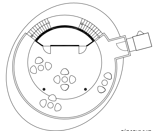
PŮDORYS 5.NP
