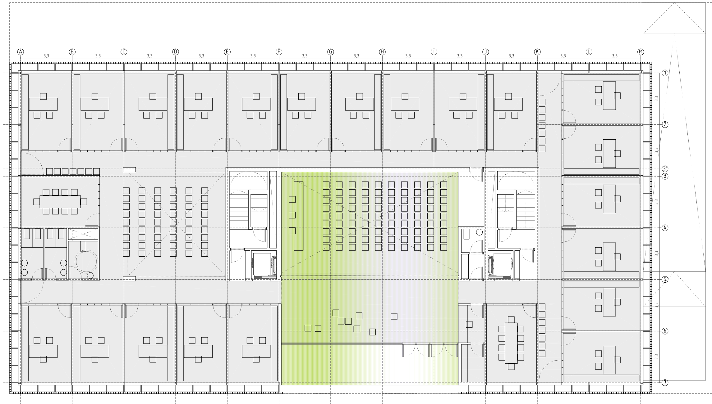
E 1:150 PLANTA BAJA
