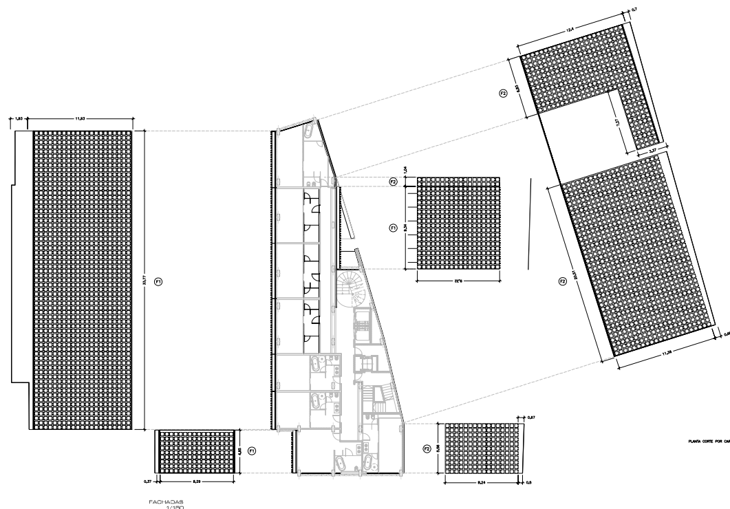
FACHADAS 1/100
