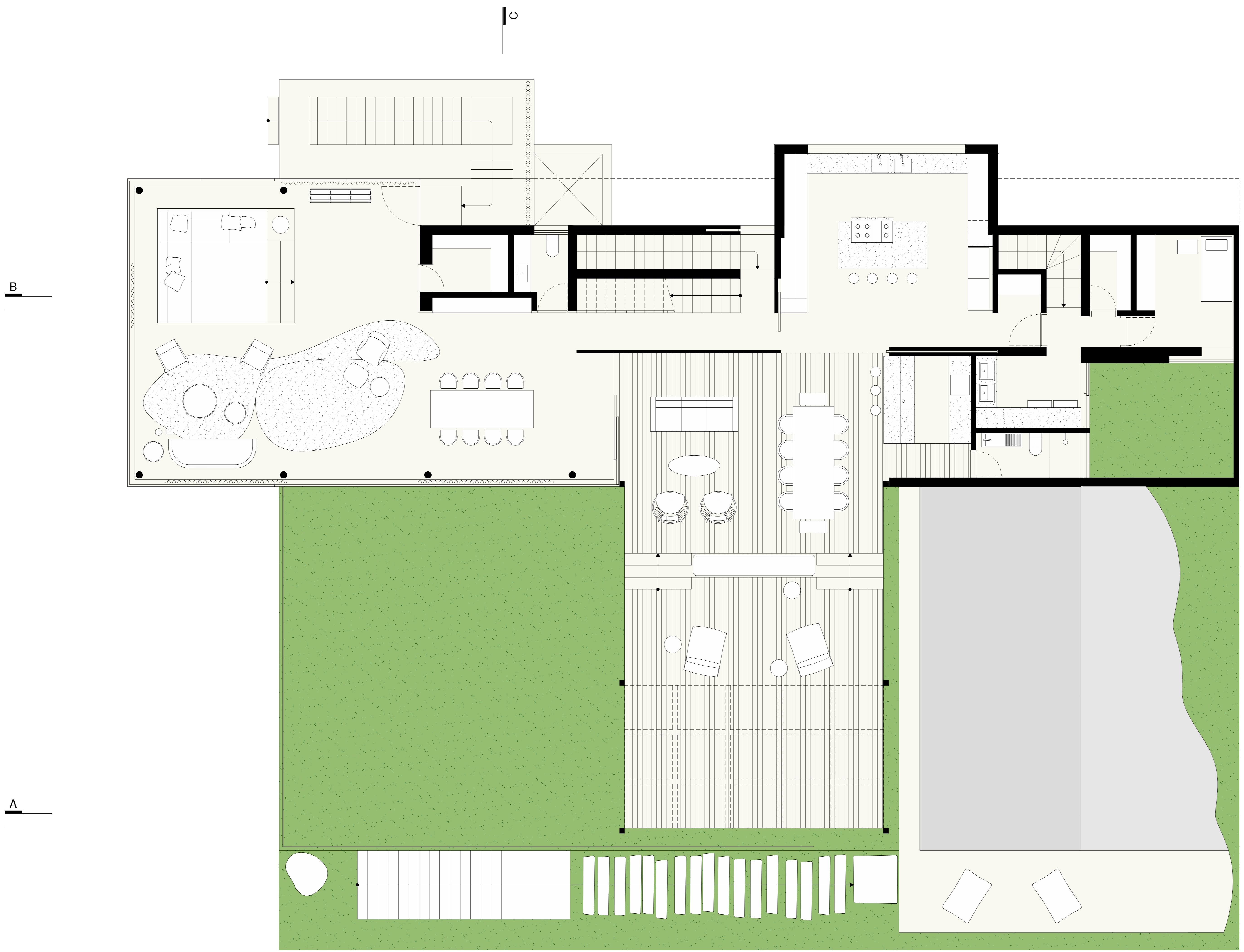
PLANTA 3° PAVIMENTO
