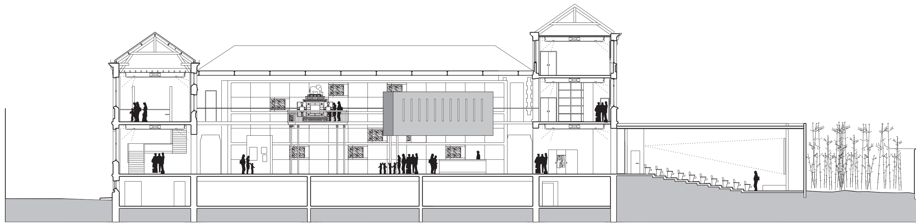
Coupe Est Ouest sur halle et réserves
